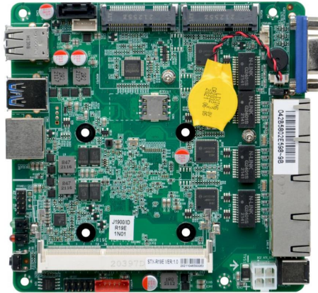
STX-R19E VER:1.0 主板正面图
