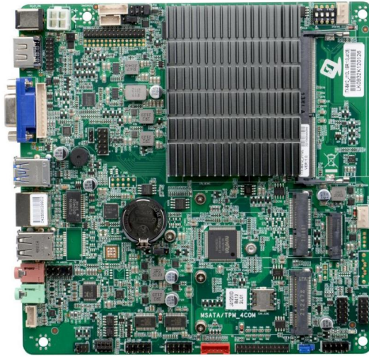
ITX-B412_J112L VER:1.0 主板正面图
