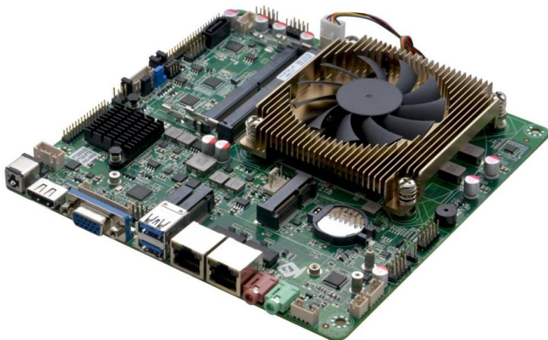
ITX-FT20 VER:1.1 主板侧面图
