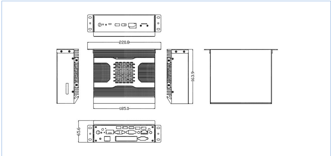
P6760F-P4尺寸图
